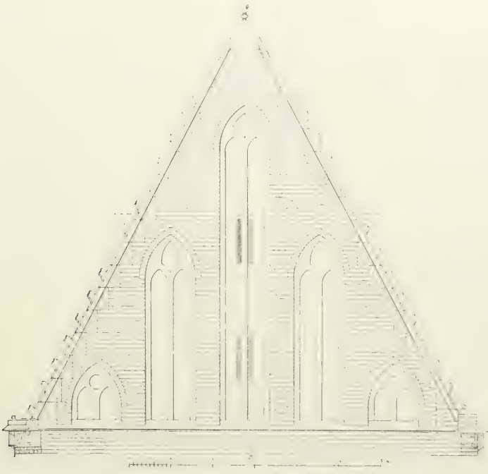
Fig. 05. Ściana szczytowa wschodnia.
